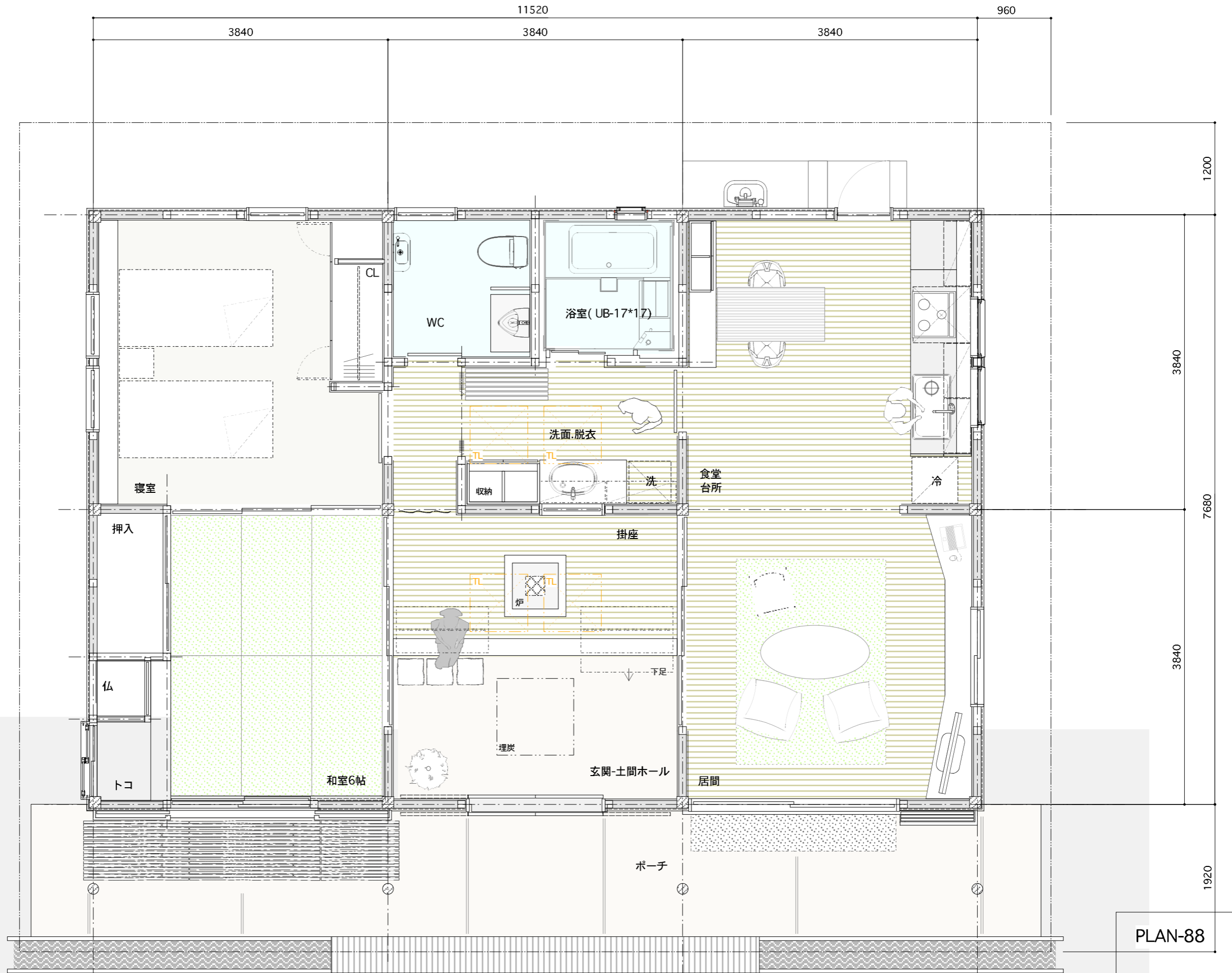
平面計画図 S=1; 50
